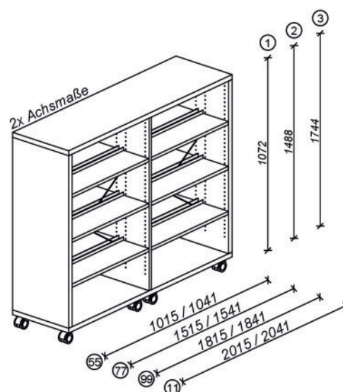
Nova Wood 25 & Nova Wood 38 Gesamthöhe
