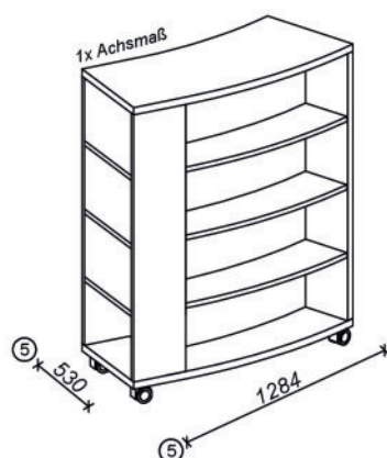
Nova Rund 38 Mobile Ausführung mit Stirnseiten Regal Bemaßungen
