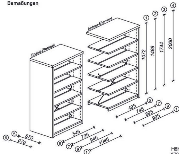
Gesamthöhe inkl. Abdeckplatte 38 mm
