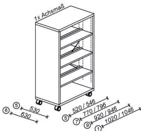
Gesamtlänge für Nova Wood 25 & Nova Wood 38 1x Achsmaß & 2x Achsmaße
