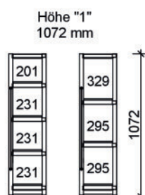
Gesamthöhe
