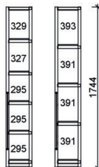
Höhe "3" 1744 mm
