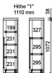
Gesamthöhe inkl. Abdeckplatte 38 mm
