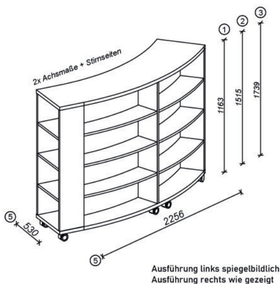
Nova Rund 38 Mobile Gesamthöhe
