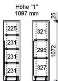
Gesamthöhe inkl. Abdeckplatte 25 mm
