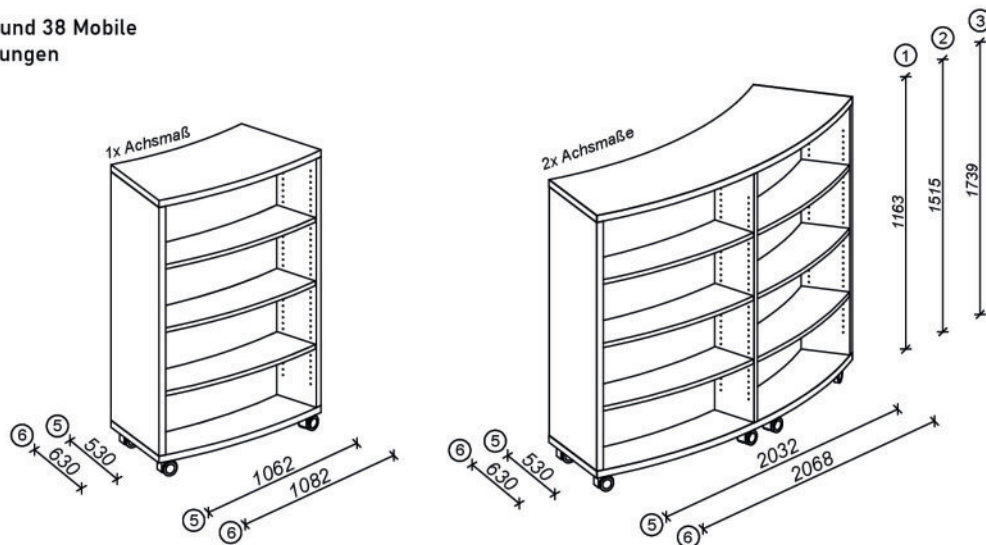
Gesamtlänge für Nova Rund 38 1x Achsmaß & 2x Achsmaße
