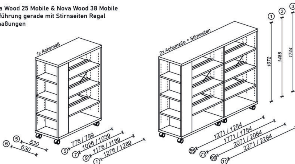
Gesamtlänge für Nova Wood 25 & Nova Wood 38 1x Achsmaß & 2x Achsmaße
