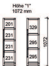
Gesamthöhe
