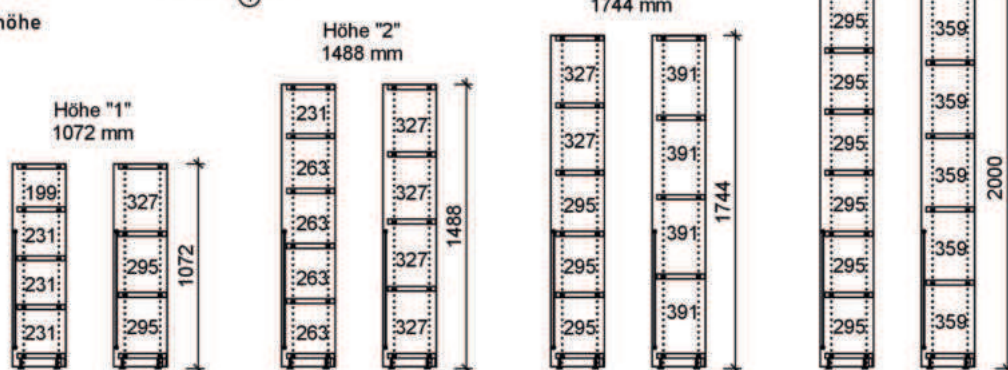
Gesamthöhe
