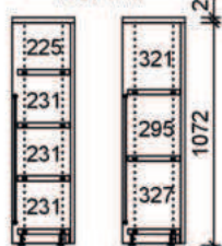
Höhe "1" 1097 mm
