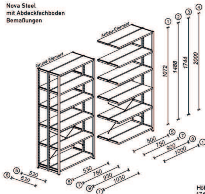
Gesamthöhe
