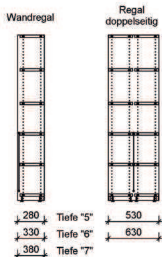
NW 25 - Ausführung - Tiefe
