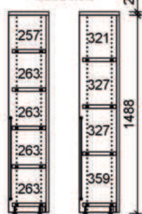
Höhe "2" 1513 mm
