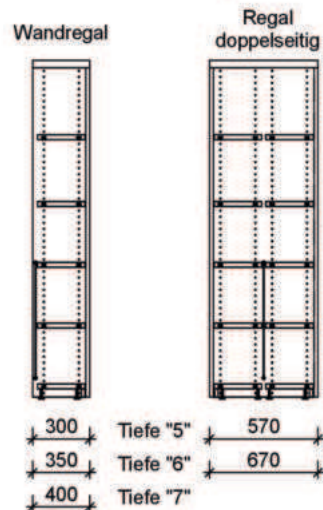
NW 38 - Ausführung - Tiefe
